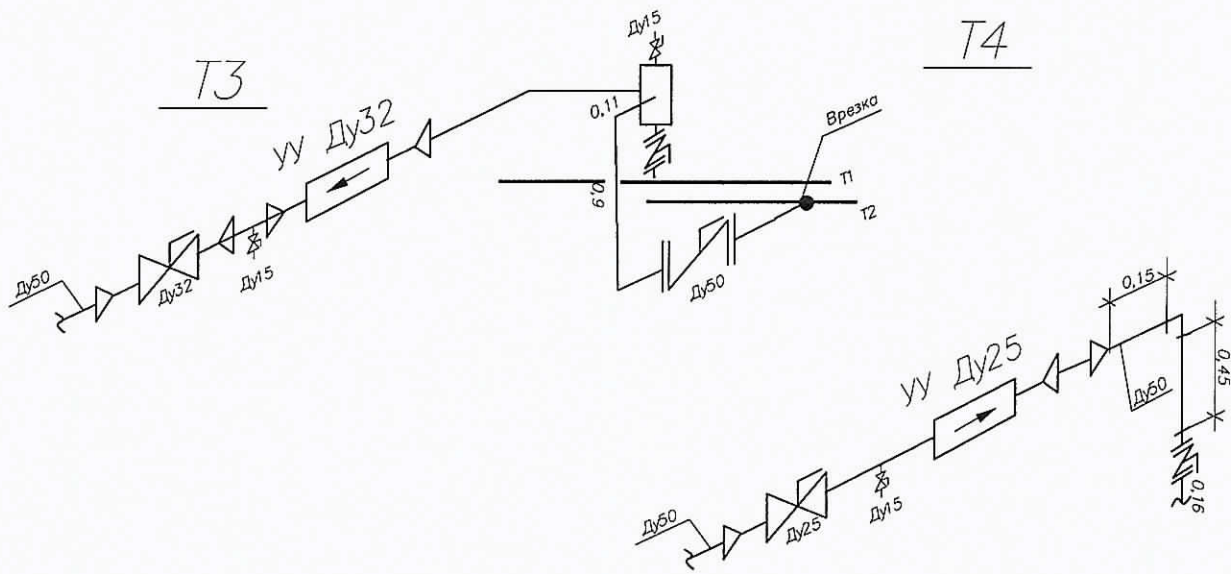
Аксонметрическая схема
