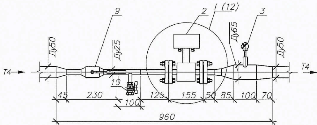
Аксонметрическая схема
